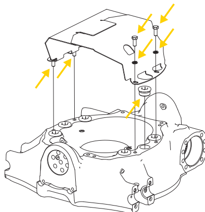
Afbeelding34. Demonstreer de beschermkap.
