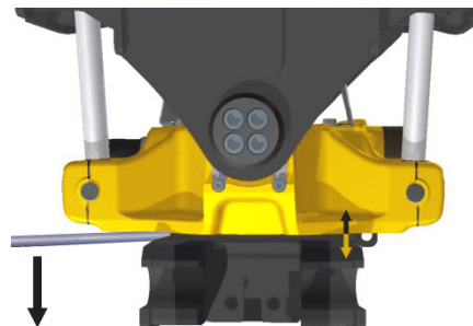
Afbeelding35. Vrij oppervlak zonder schroefkop.
