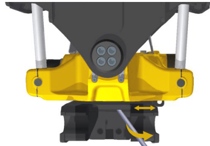
Afbeelding39. Draai de snelwissel naar rechts.
